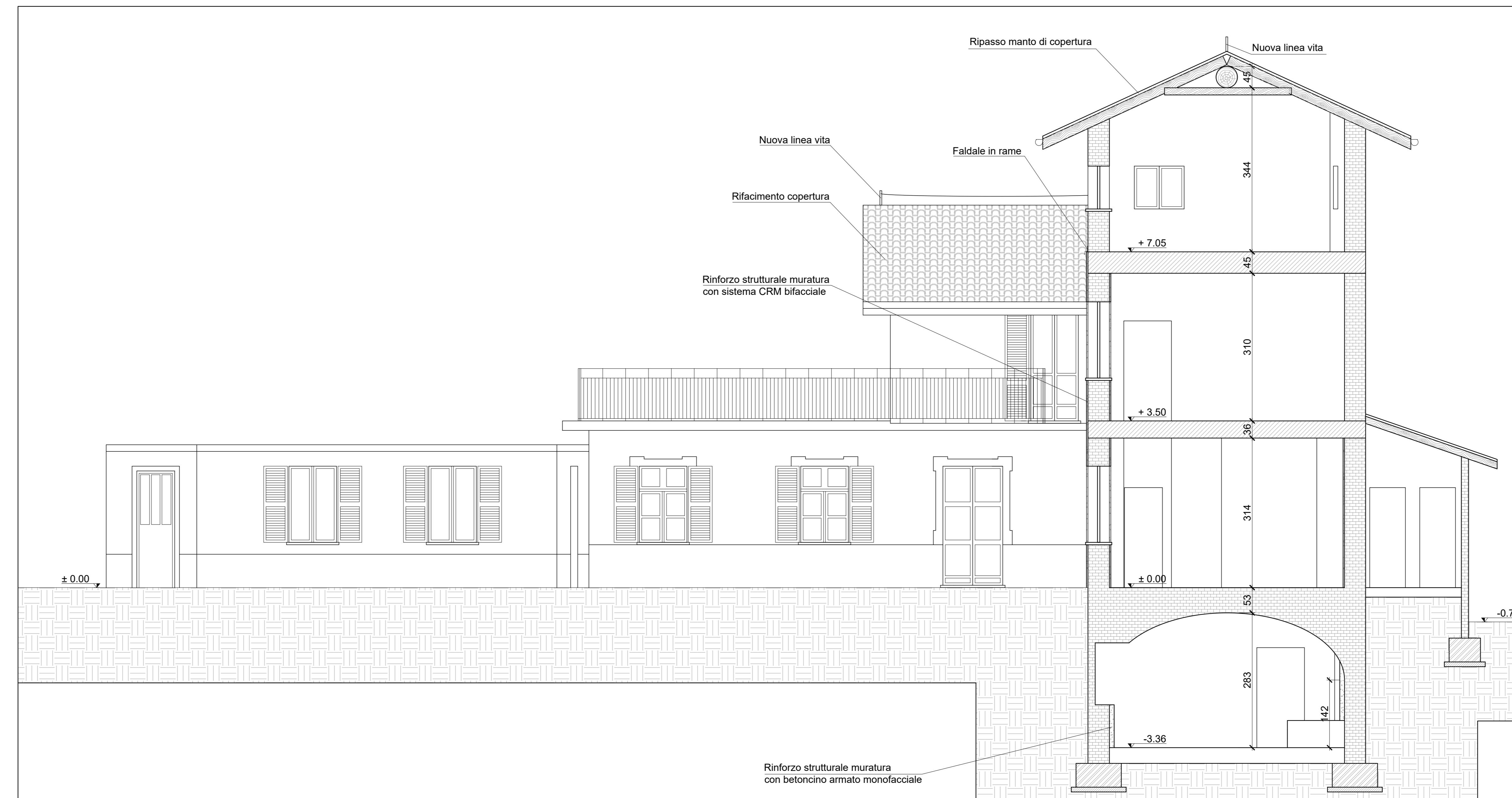
SEZIONE C-C Scala 1:50
